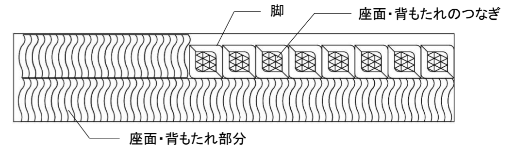
CLT切り出し図 (長さ)6,000mm (幅)1,200mm (厚さ)90mm
