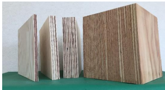
厚さ(左から)12mm、24mm、50mm、200mm
