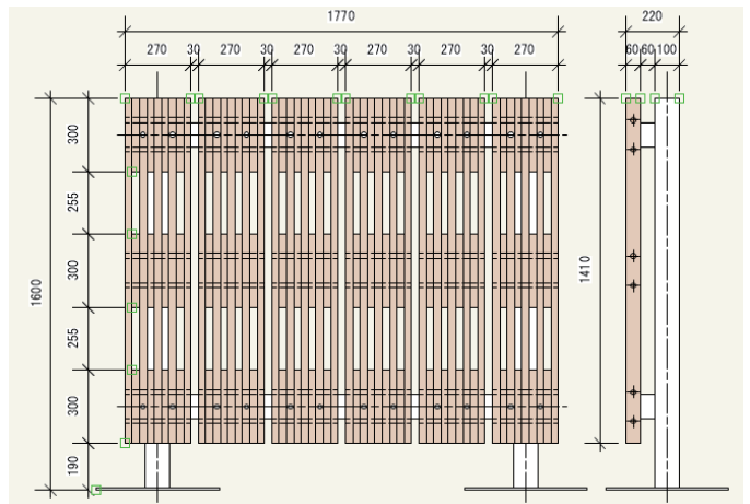
タテ棧タイプ
