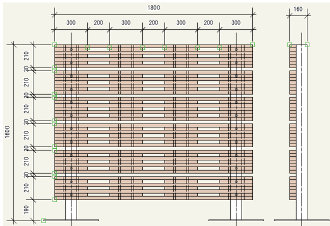
ヨコ棧タイプ
